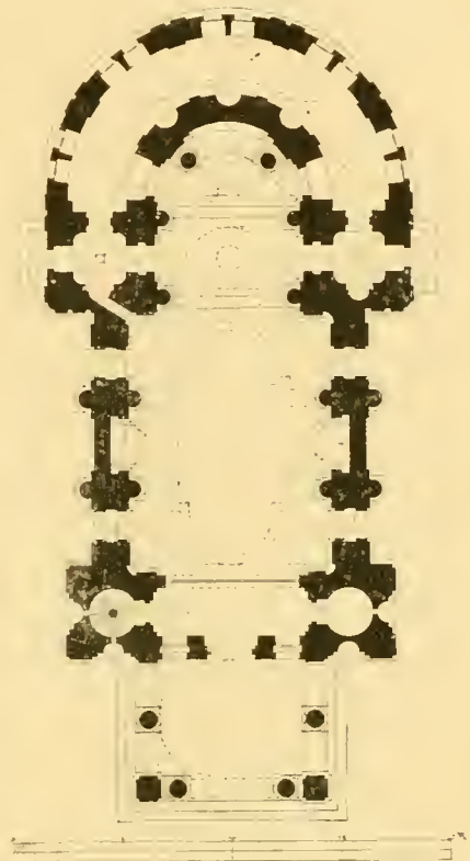
Fig. 82. Johanneskirche zu Innsbruck. Grundriss.
